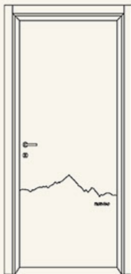
MONVISO
