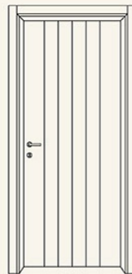
P56 B
